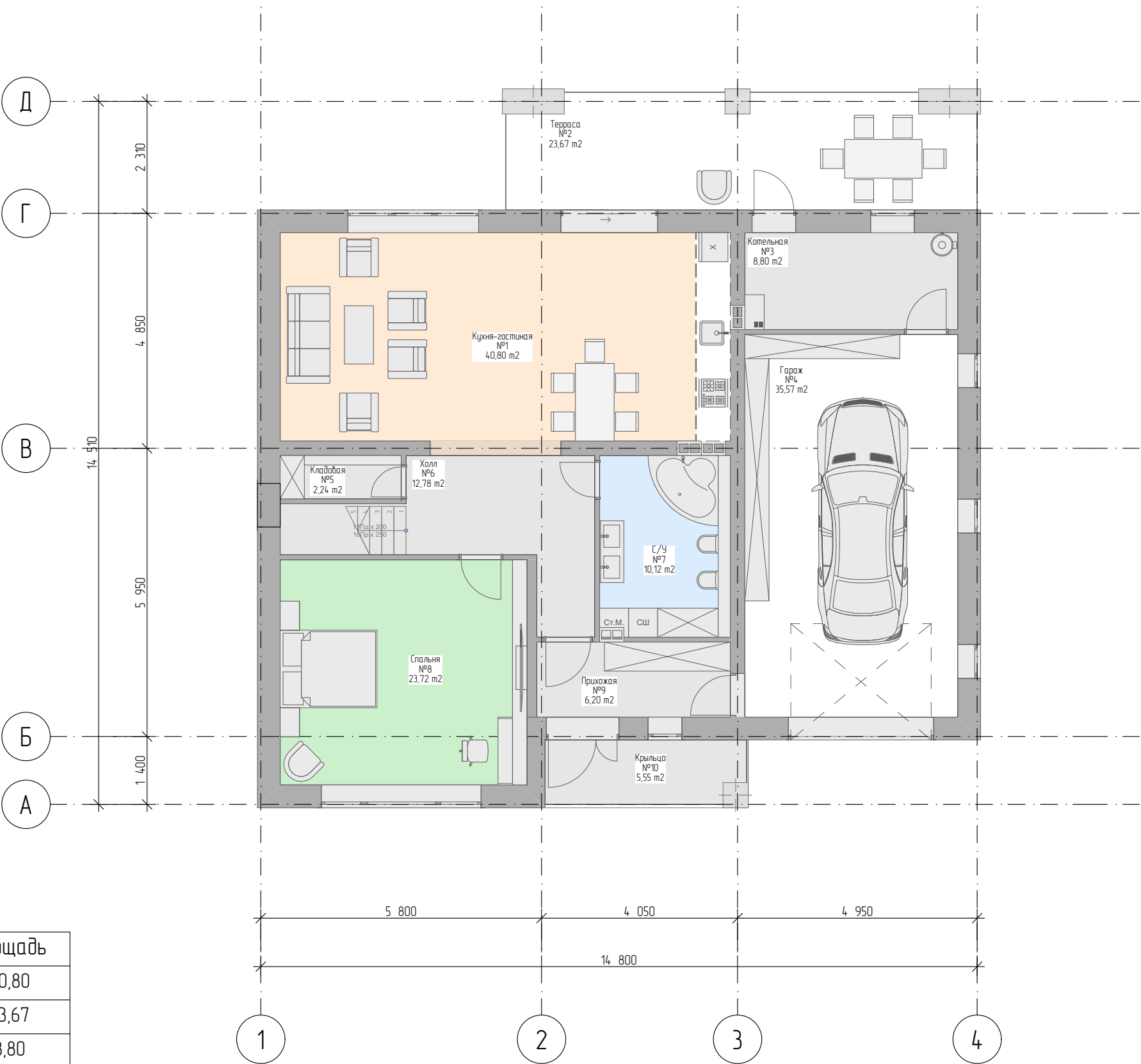
План расположения зон первого этажа М1:100
