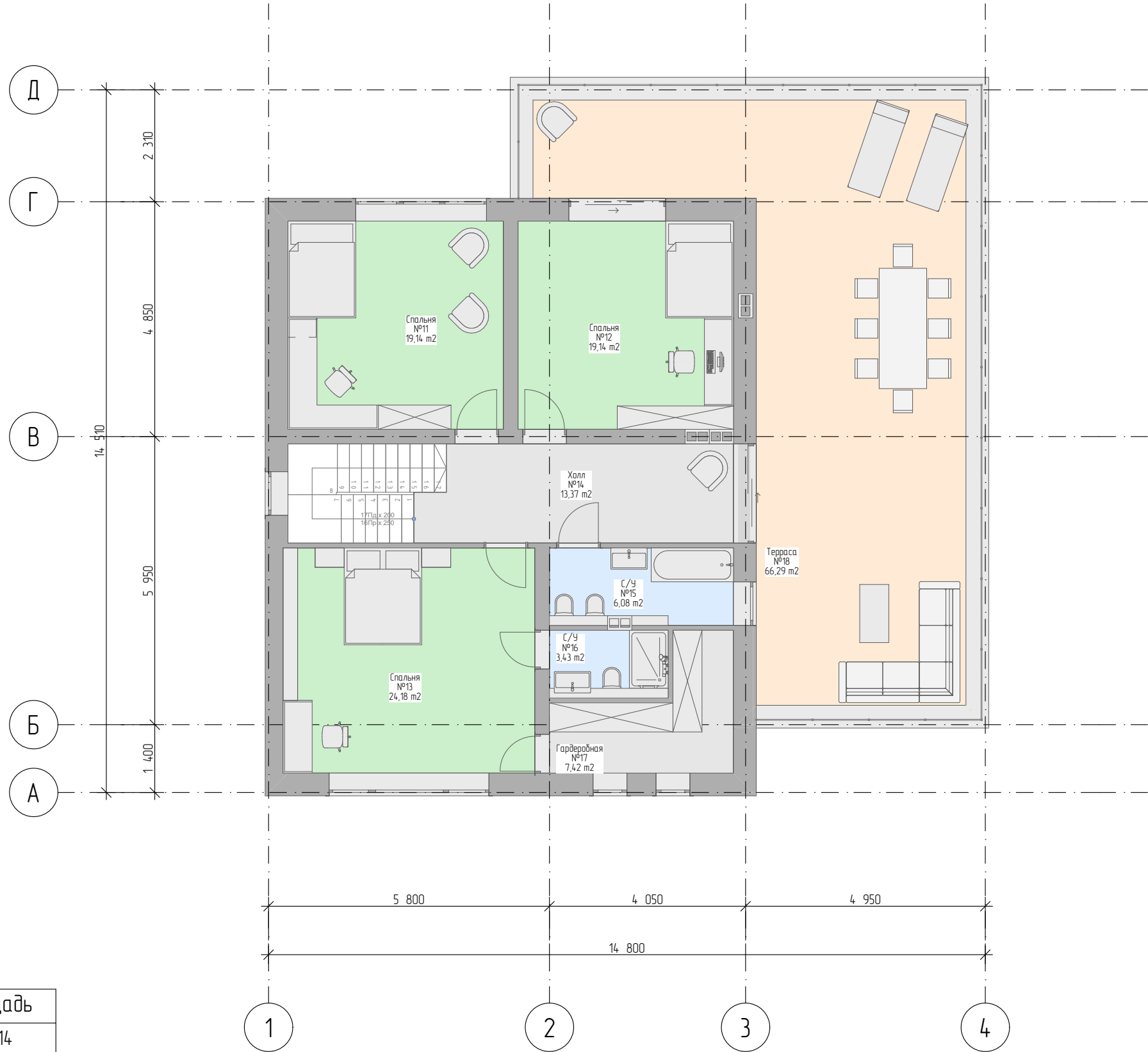
План расположения зон второго этажа М1:100
