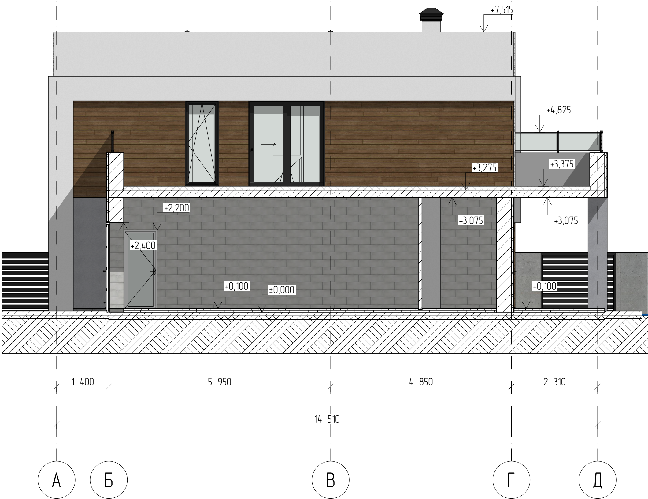
Разрез 3-3 М1:60
