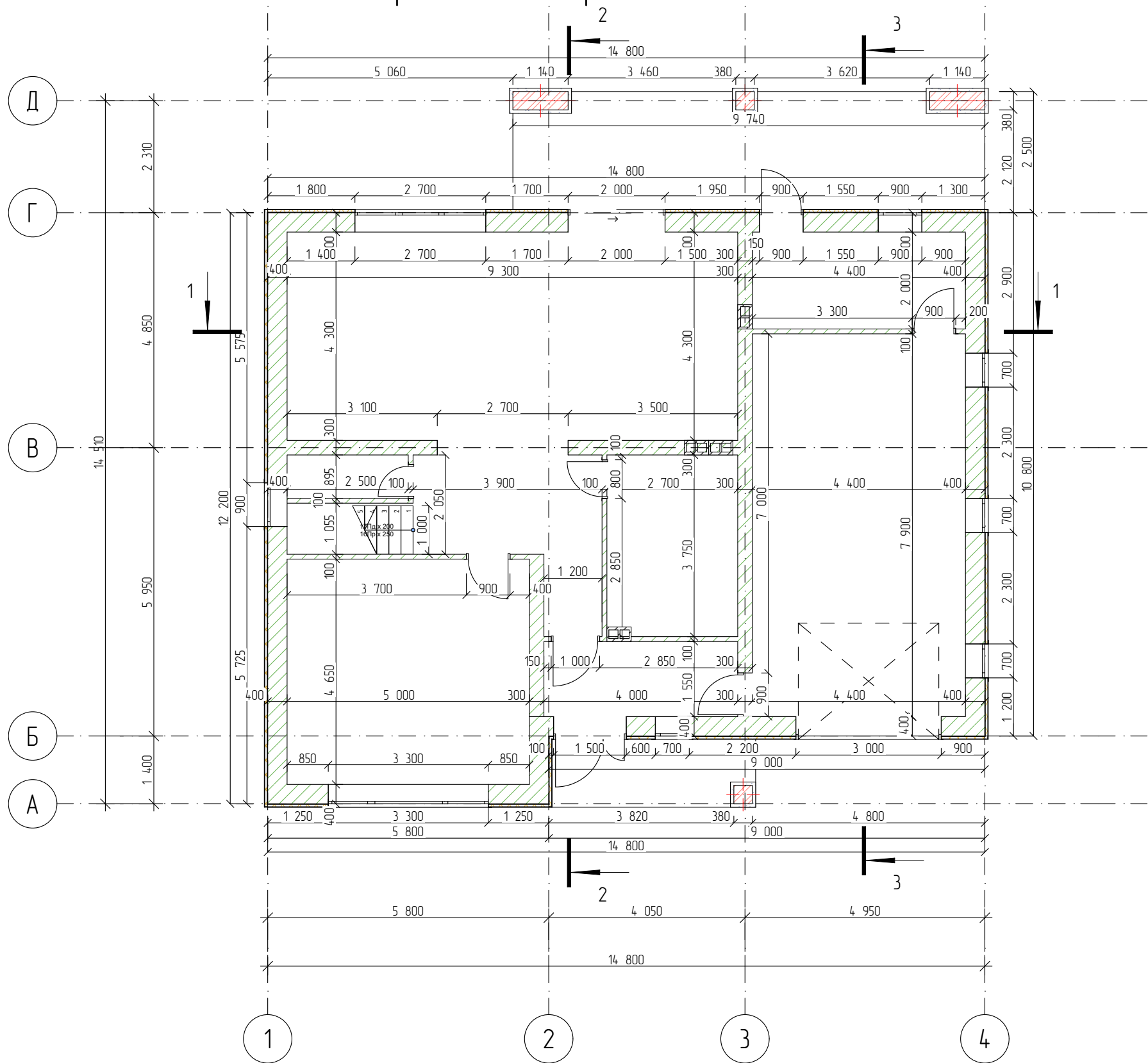
Обмерочный план первого этажа М1:100
