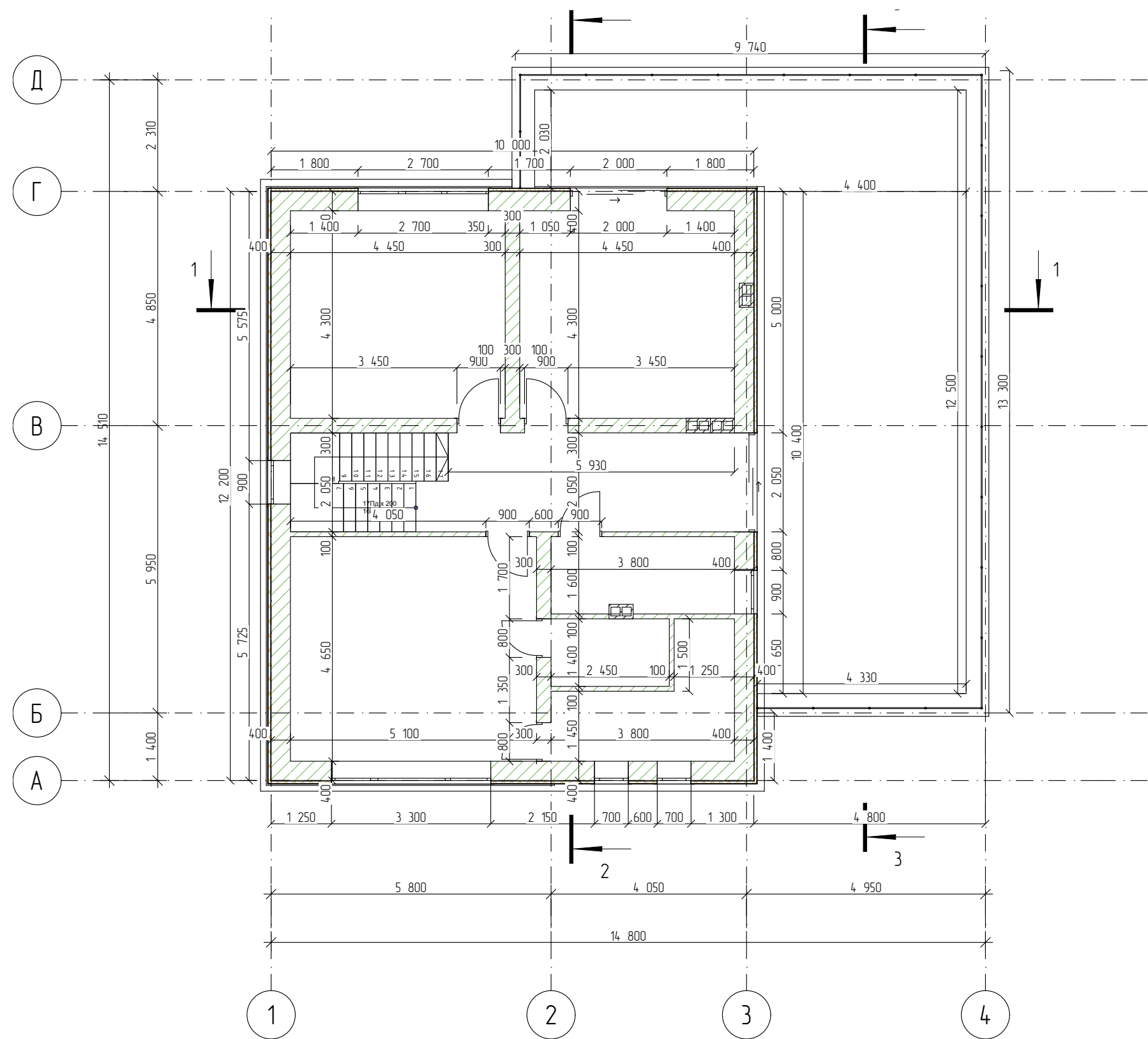
Обмерочный план второго этажа М1:100
